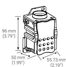
UD-400112AL & UD-400112CU 400 A – IEC 335 A – cULus 1 câble – 12 câbles
