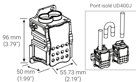
UD-400212AL & UD-400212CU 400 A – IEC 400 A – cULus 2 câbles – 12 câbles
