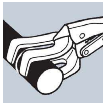
42 24 280 Mâchoires en acier coulé thermorésistant maintient centrés les tubes ou les pièces rondes les unes à côté des autres lors du soudage
