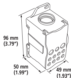
Connecteur FLG 400 A avec ERIFLEX FLEXIBAR
