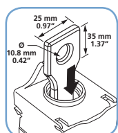
Liaison directe du répartiteur à l'appareillage
