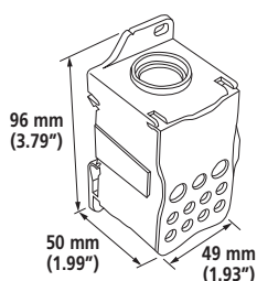
Connecteur FLG 250 A avec ERIFLEX FLEXIBAR
